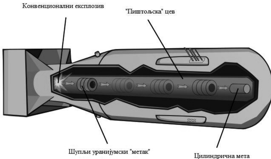
Слика 1: Модел „пиштољ” бомбе
